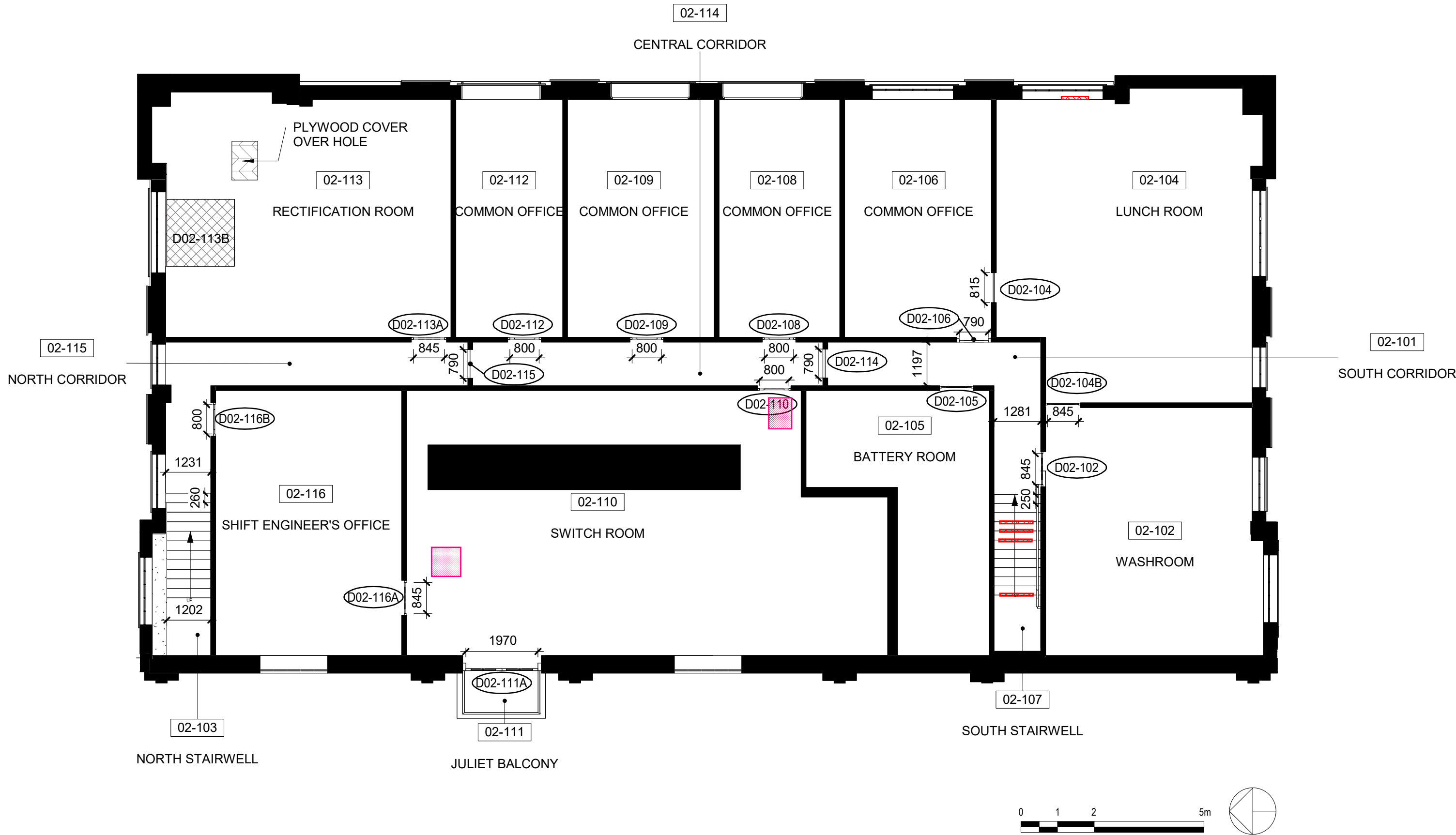
1 02 - SWITCH HOUSE 1 : 100
