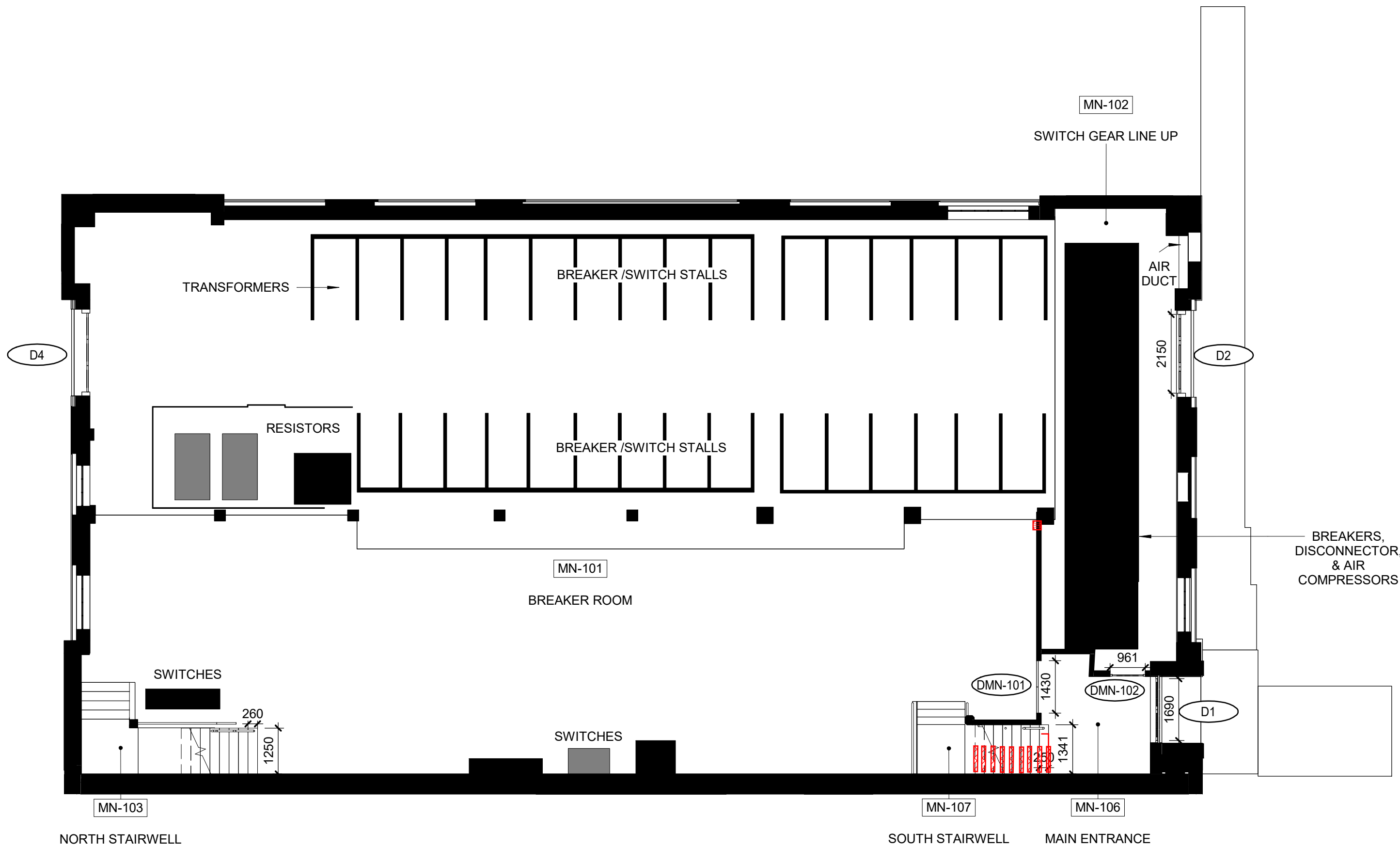
1 BM - SWITCH HOUSE 1 : 100
