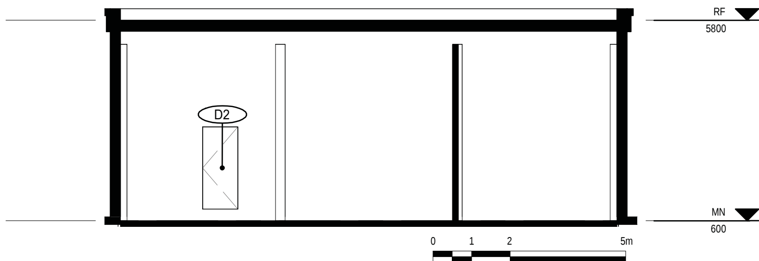
6 MN_SOUTH 1 : 100
