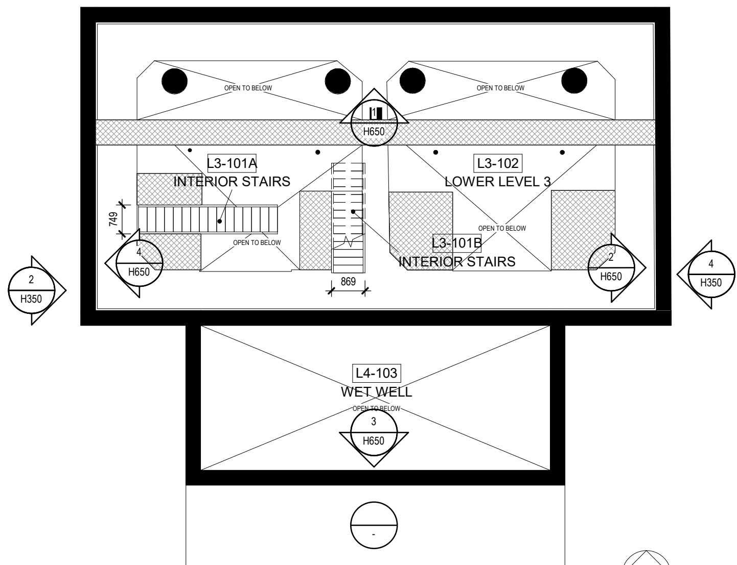
4 LOWER 3 1 : 100
